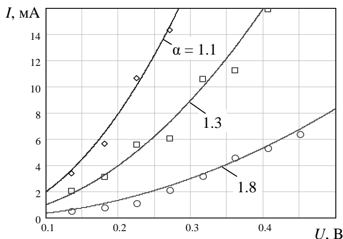
Рис. 5.3. Вольт-амперные характеристики диодов: \diamond – германий, \square – легированный кремний, \circ – арсенид галлия
