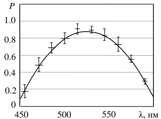
Рис. 5.5. Зависимость степени поляризации света от длины волны
