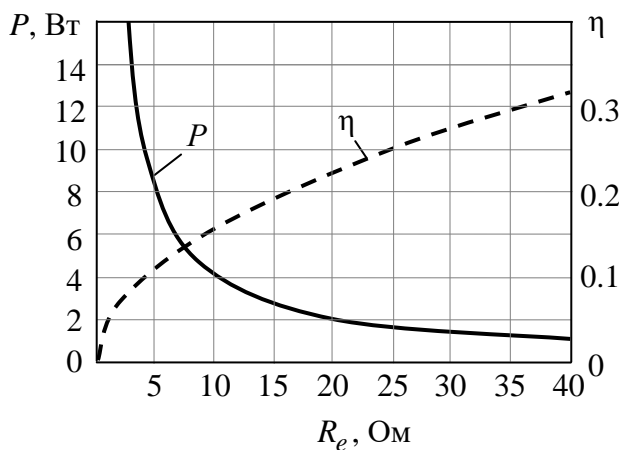
Рис. 5.4. Зависимость мощности и КПД от сопротивления нагрузки
