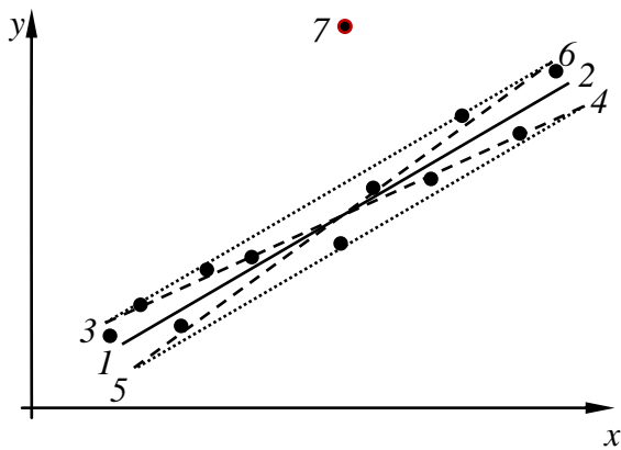
Рис. 4.3. Построение прямых для определения параметров линейной зависимости по графику
