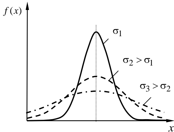
Рис. 2.3. Нормальное распределение
