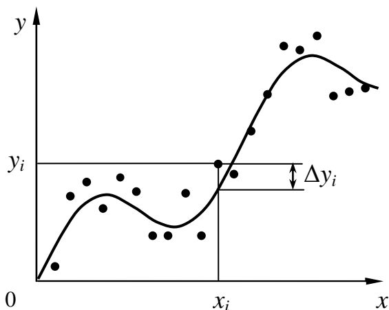
Рис. 4.1. Регрессионная кривая
