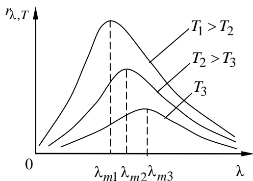
Рис. 5.1. Зависимость спектральной лучеиспускательной способности от длины волны
