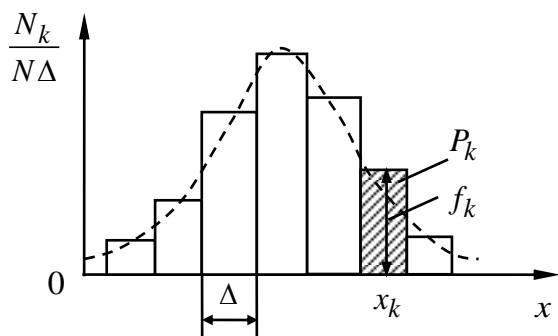
Рис. 2.1. Гистограмма
